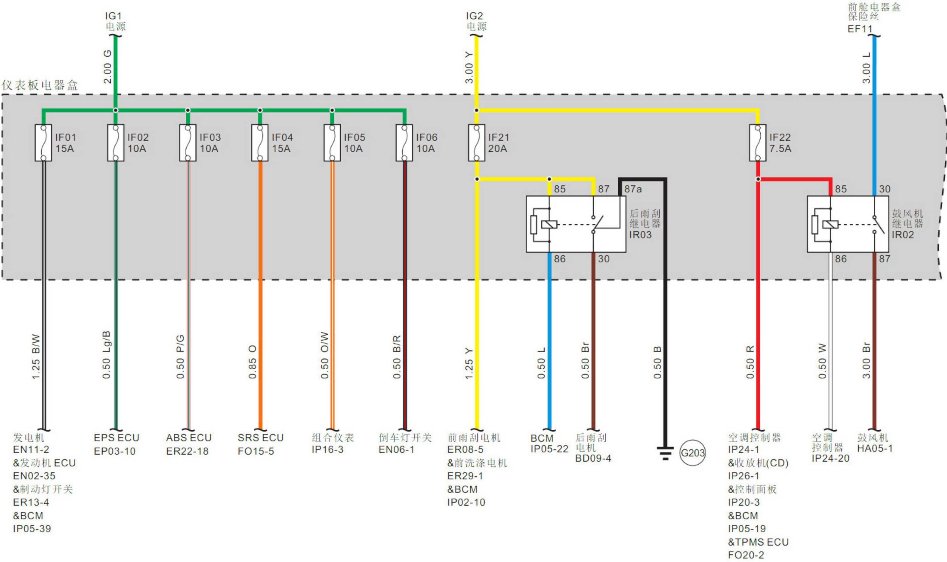
仪表板电器盒电源分配 (二)
