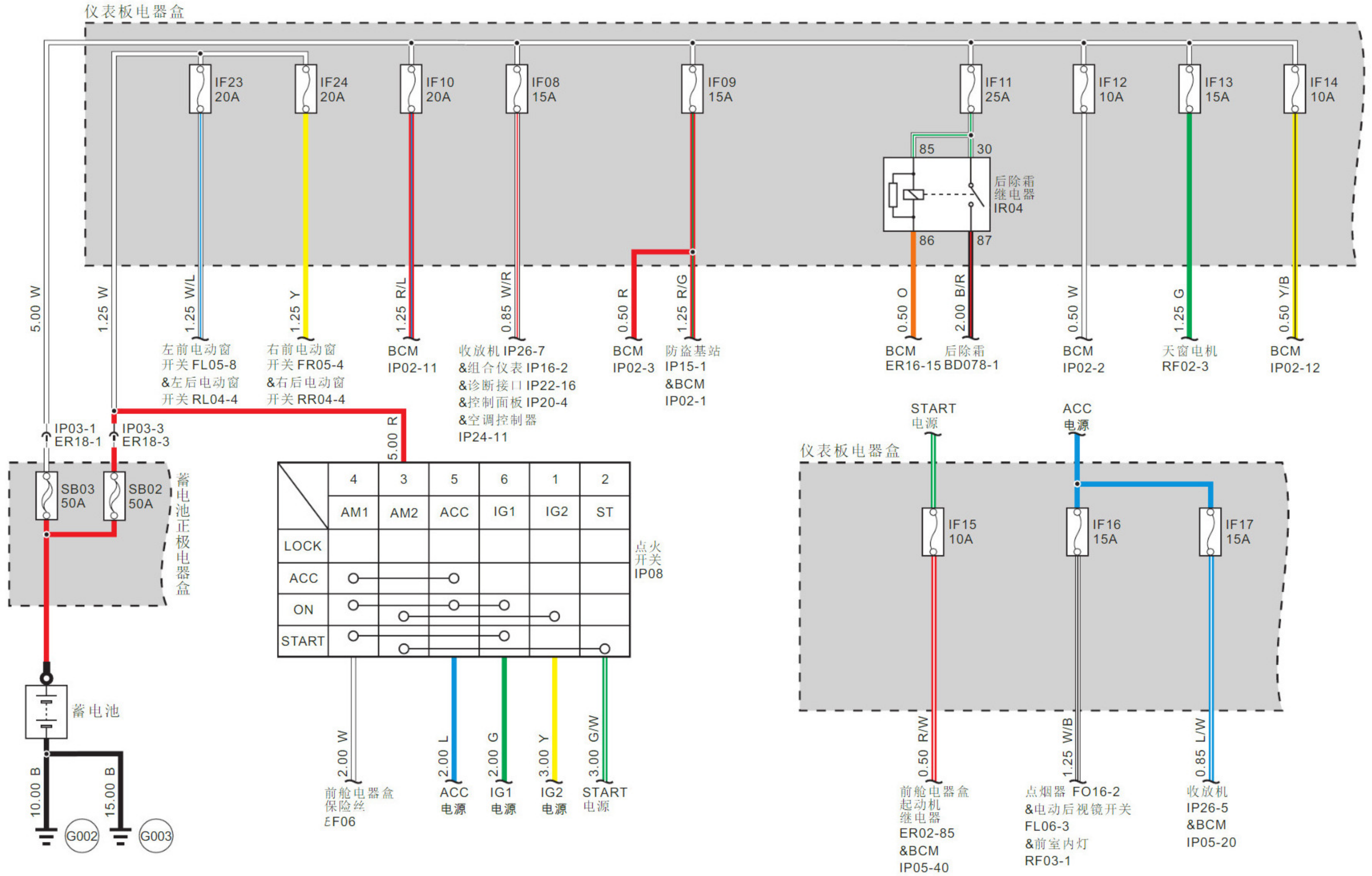
仪表板电器盒电源分配(一)
